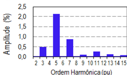
Espectro Harmônico de Tensão (Valores Médios)
